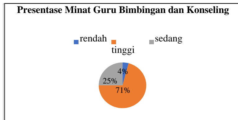
Gambar 2. Diagram Pie Hasil Persentase Kategorisasian Hasil Pengukuran
