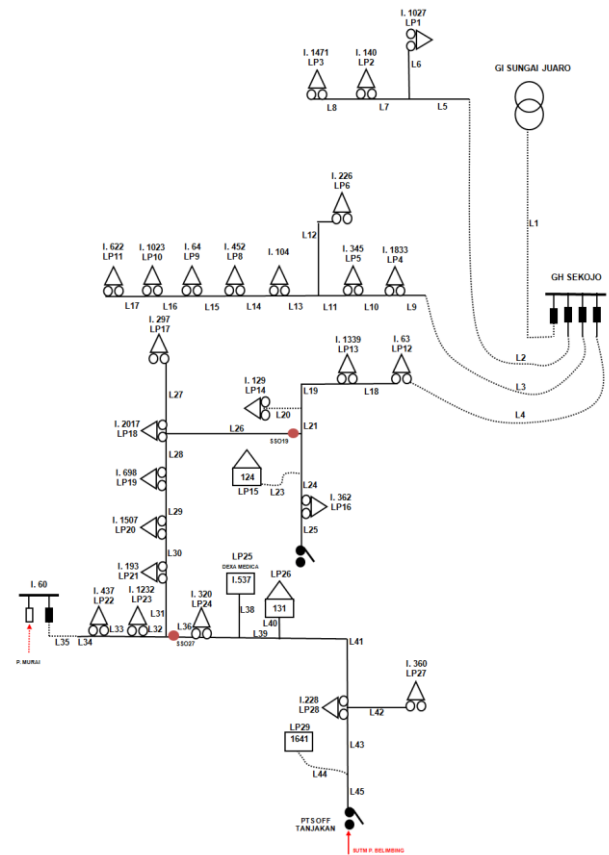
Gambar 5. Lokasi penempatan sectionalizer yang dipilih
