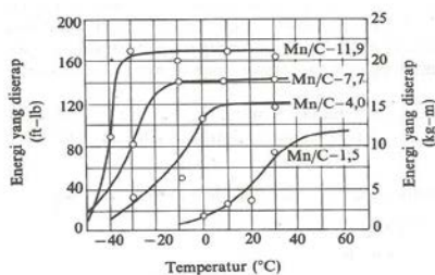
Gambar 1: Pengaruh perbandingan Mn/C terhadap kurva transisi
