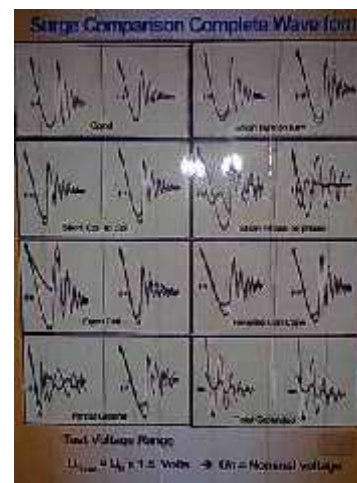
Gambar 2.1 referensi bentuk gelombang surge tester
