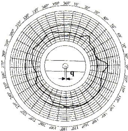
Gambar 13. Grafik kebulatan pengukuran posisi 1 (1 skala dalam grafik = 1 \mu\text{m} )
