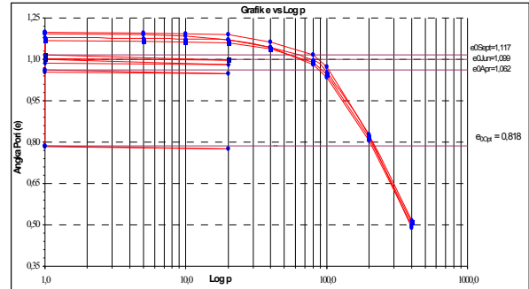
Gambar 4.2.2. Tekanan Pengembangan Lokasi Km. 20
