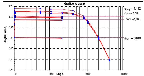
Gambar 4.2.3. Tekanan Pengembangan Lokasi Km. 30
