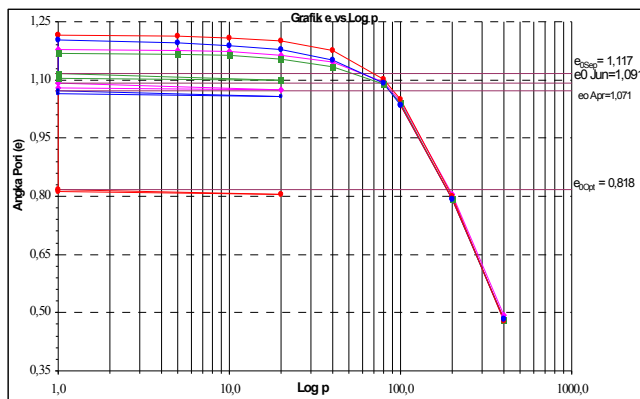
Gambar 4.2.1. Tekanan Pengembangan Lokasi Km.10
