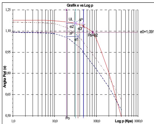
Gambar 4.6.2. Grafik Total Heave Pada lokasi Km. 10 Bulan Juni
