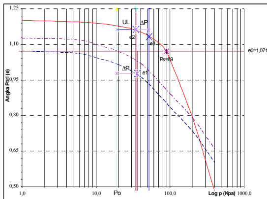
Gambar 4.6.1. Grafik Total Heave Pada lokasi Km. 10 Bulan April
