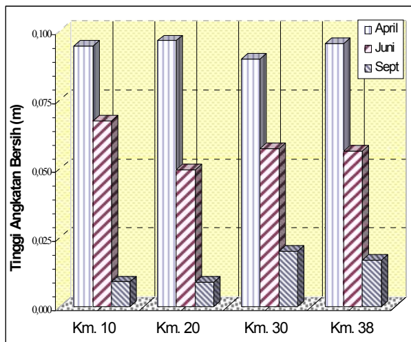
Gambar 4.7. Grafik Perbedaan Total Heave
