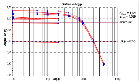
Gambar 4.2.4. Tekanan Pengembangan Lokasi Km. 38
