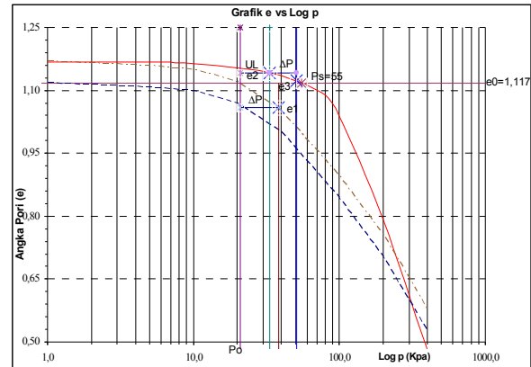
Gambar 4.6.3. Grafik Total Heave Pada Lokasi Km. 10 Bulan September
