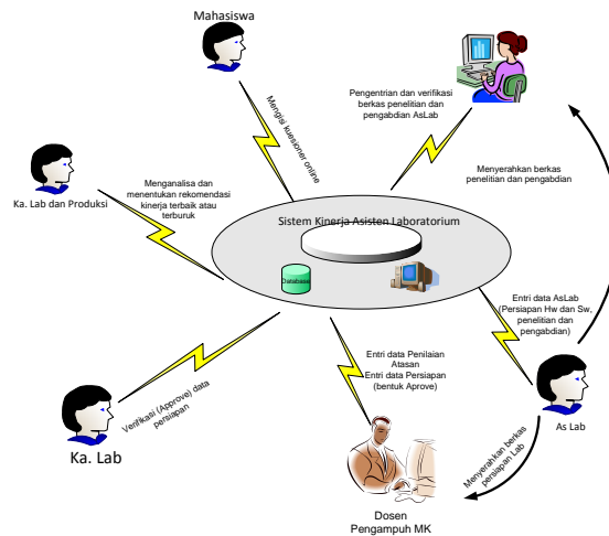
Gambar 1. Perancangan Arsitektur SPK Kinerja Asisten Laboratorium
