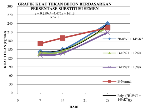
Gambar IV.10. Grafik Hubungan Kuat Tekan Beton dengan Persentase Campuran Abu Ampas Tebu dan Abu Cangkang Kerang Terhadap Umur 7,14 dan 28 hari
