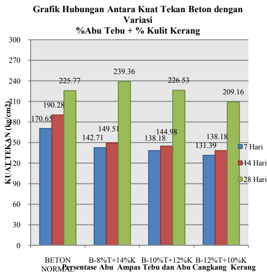
Gambar IV.9. Diagram Hubungan Kuat Tekan Beton dengan Persentase Campuran Abu Ampas Tebu dan Abu Cangkang Kerang Terhadap Umur 7,14 dan 28 hari
