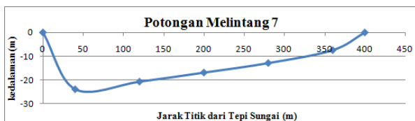
Gambar IV.4. Grafik kedalaman terhadap jarak pada potongan melintang 7
