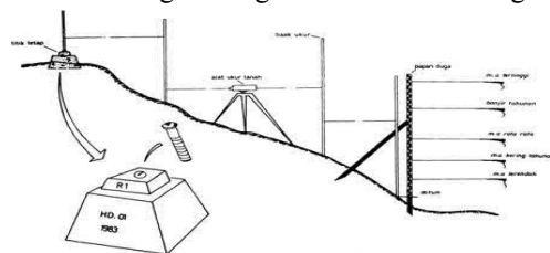
Sumber : Perencanaan Bangunan Pantai, 2012 Gambar II.1. Sketsa Pengukuran Datum Tinggi Muka Air
