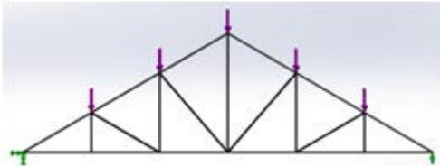
Gambar 3.6 Pembebanan Sampel
