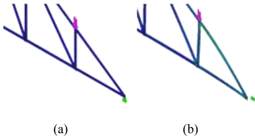
Gambar 4.4 Proses Keruntuhan Rangka Tipe Pratt (L = 12 Meter) (a) Sebelum mendapat beban berlebihan (b) Setelah mendapat beban berlebihan
