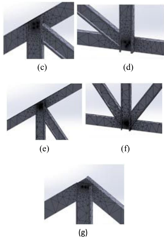
Gambar 4.2 Hasil Meshing Tiap Simpul Pada Tipe Howe, (a) simpul 1, (b) simpul 2, (c) simpul 3, (d) simpul 4, (e) simpul 5, (f) simpul 6, (g) simpul 7
