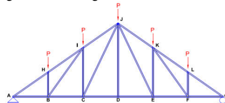
Gambar 3.4 Tipe Pratt
