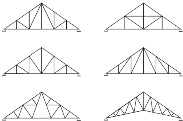
Gambar 2.1 Bentuk Rangka Atap
