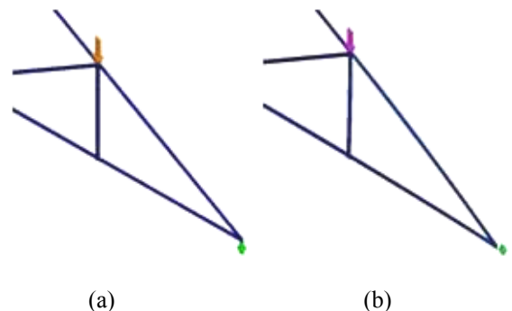
Gambar 4.10 Proses Keruntuhan Rangka Tipe Howe (L = 24 Meter) (a) Sebelum mendapat beban berlebihan (b) Setelah mendapat beban berlebihan
