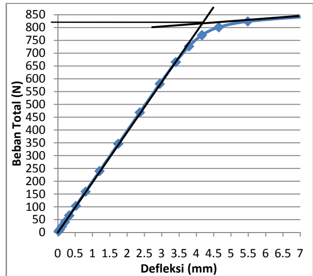
Grafik 4.2 Beban – Defleksi Tipe Howe Bentang Teoritis 24 meter
