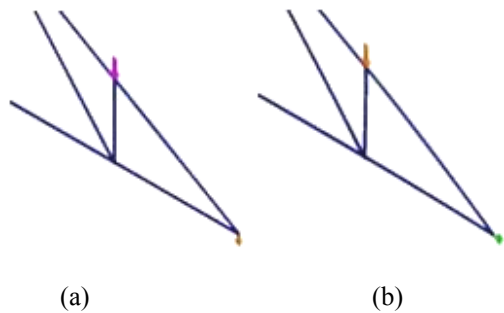
Gambar 4.6 Proses Keruntuhan Rangka Tipe Pratt (L = 24 Meter) (a) Sebelum mendapat beban berlebihan (b) Setelah mendapat beban berlebihan
