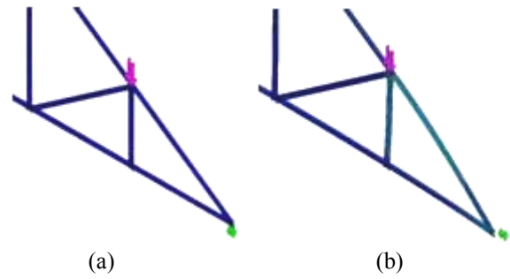
Gambar 4.8 Proses Keruntuhan Rangka Tipe Howe (L = 12 Meter) (a) Sebelum mendapat beban berlebihan (b) Setelah mendapat beban berlebihan
