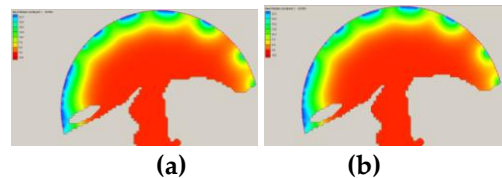
Gambar 18. Model Pola Salinitas Time Step 60 (Surut terendah), (a) Tanpa Pengaruh Angin; (b) Pengaruh angin
