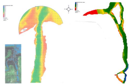
Gambar 10. Model Pola Arus Time Step 328 (MSL menuju pasang tertinggi)
