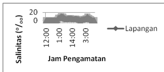
Gambar 14. Grafik Verifikasi Salinitas (22 – 24 Juli 2011)
