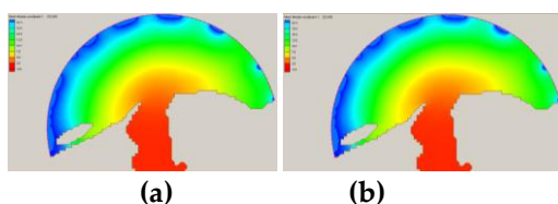
Gambar 16. Model Pola Salinitas Time Step 332 (Pasang tertinggi), (a) Tanpa Pengaruh Angin; (b) Pengaruh angin
