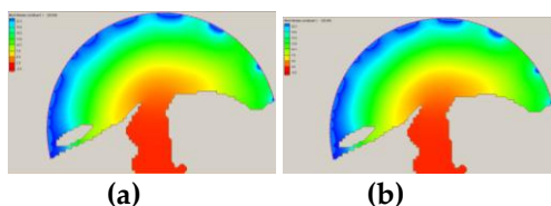
Gambar 15. Model Pola Salinitas Time Step 328 (MSL menuju pasang tertinggi), (a) Tanpa Pengaruh Angin; (b) Pengaruh angin
