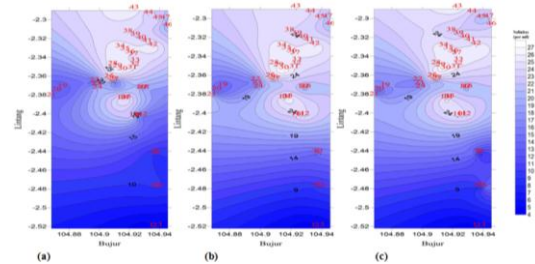
Gambar 7. Grafik Salinitas pada Kondisi Surut (a) 0,2 D; (b) 0,5 D; (c) 0,8 D
