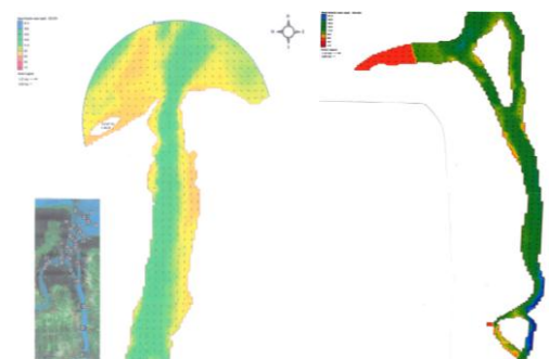
Gambar 11. Model Pola Arus Time Step 332 (Pasang tertinggi)
