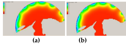
Gambar 17. Model Pola Salinitas Time Step 56 (MSL menuju surut terendah), (a) Tanpa Pengaruh Angin; (b) Pengaruh angin
