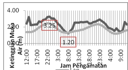
Gambar 3. Grafik Ketinggian Muka Air Laut; data prediksi: (Surbakti, 2011)
