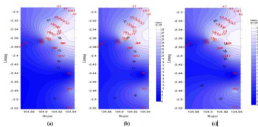
Gambar 6. Grafik Salinitas pada Kondisi Pasang (a) 0,2 D; (b) 0,5 D; (c) 0,8 D
