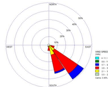
Gambar 4. Windrose kecepatan dan arah angin pada bulan Juli 2011
