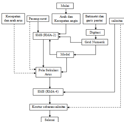
Gambar 2. Diagram alir pembuatan model pola sebaran salinitas (Ket: --- = verifikasi)
