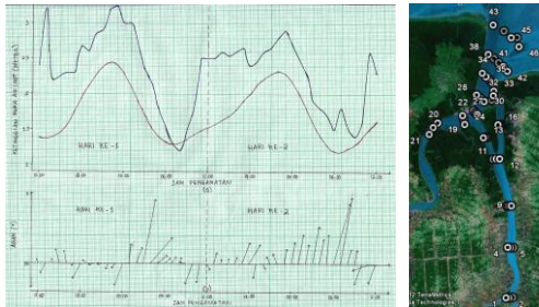
Gambar 5. Stik Plot Arus di Perairan TPI Sungsang dari 22 – 23 Juli 2011 berdasarkan kondisi pasang surut. (a) Pasang surut; (b) Arus
