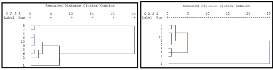
Gambar 6. Dendrogram Cu (kiri) dan Pb (kanan) terhadap skewness
