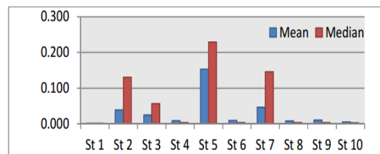
Gambar 3. Grafik mean dan median (dalam mm)
