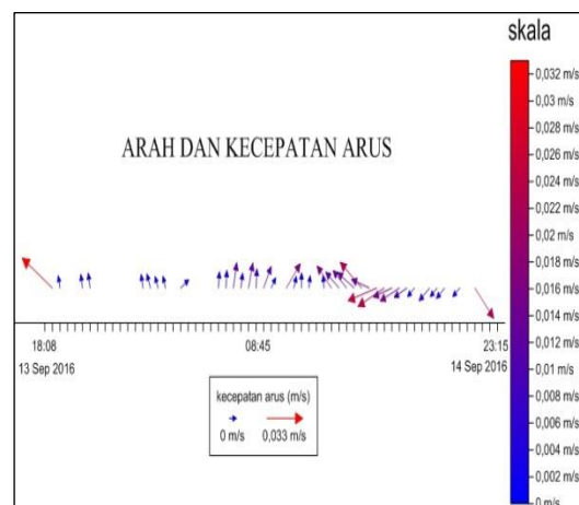
Gambar 2. Stick plot arah dan kecepatan arus Muara Sugihan.
