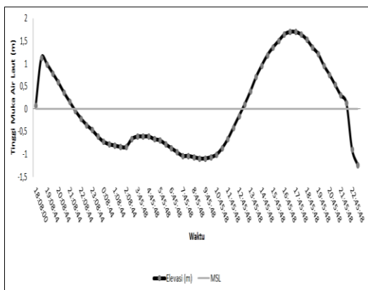
Gambar 3. Periode pasang dan surut Muara Sugihan
