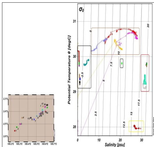
Gambar 7. Diagram T-S Kondisi Menuju Surut
