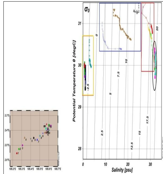
Gambar 6. Diagram T-S Kondisi Menuju Pasang
